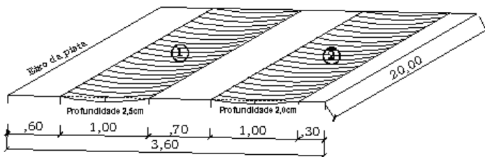
Figura 3 - Perfil das trilhas de roda.
