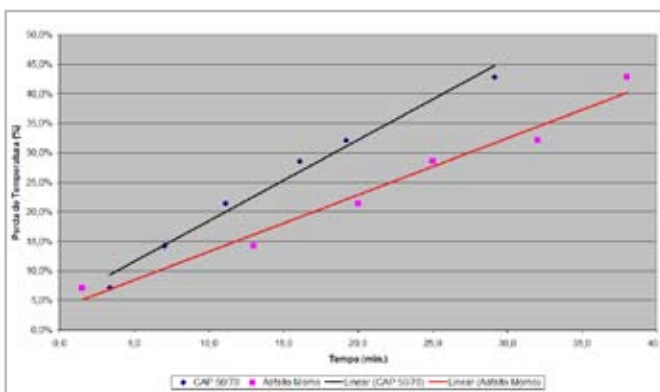
Gráfico 3 – Perda de Temperatura x Tempo
