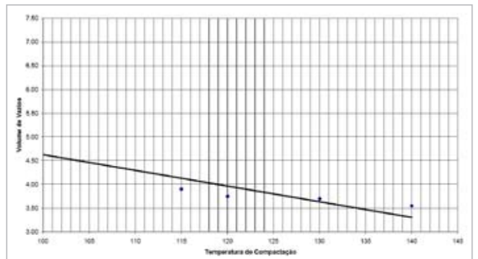
Gráfico 2 – Comportamento da Compactação do Asfalto-morno
