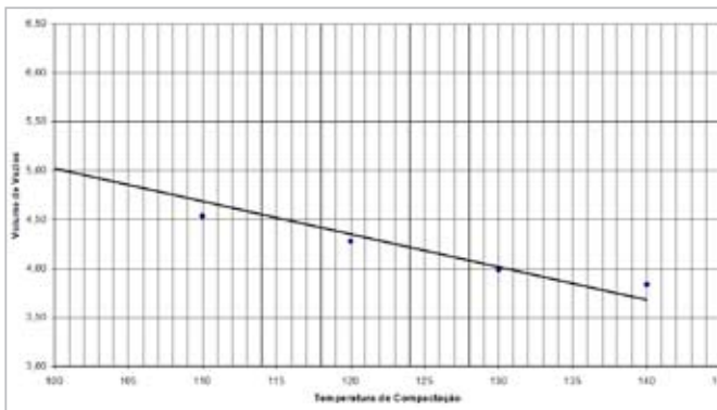
Gráfico 1 – Comportamento da Compactação do CAP 50/70
